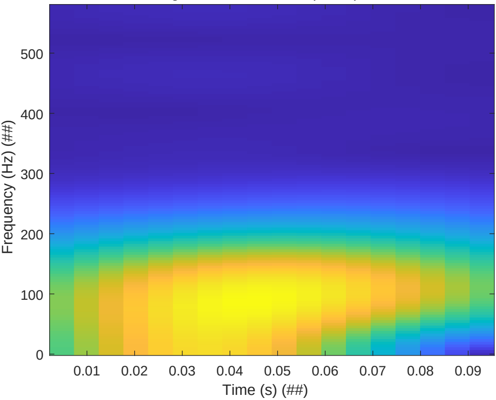
Signal: Sine-Gaussian (##-##)
